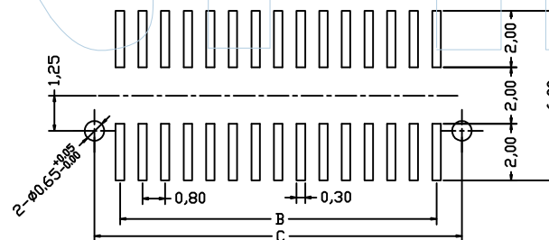
P.C.B PATTEN
