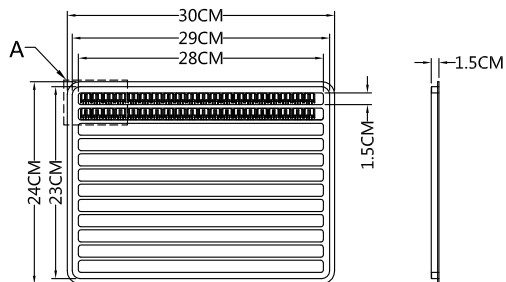
吸塑盘下盖(12格)
